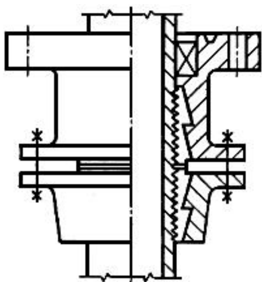
Клиньевой колонный фланец (79)
