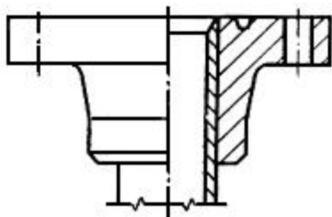
Камерная цементирующая головка (66)
