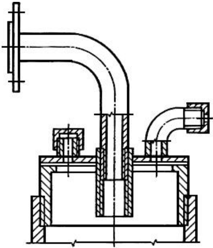
Приварной колонный фланец (77)
