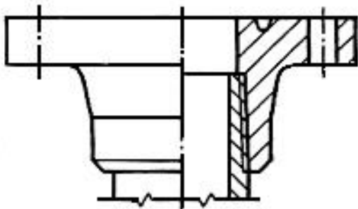
Резьбовой колонный фланец (78)
