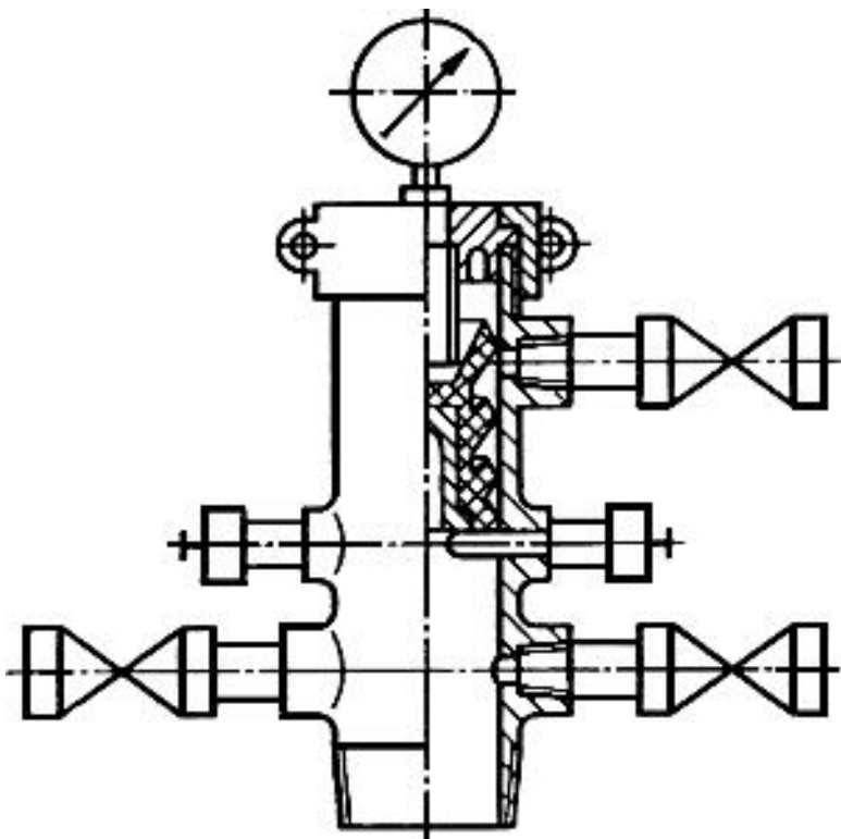
Клиньевой колонный фланец (79)
